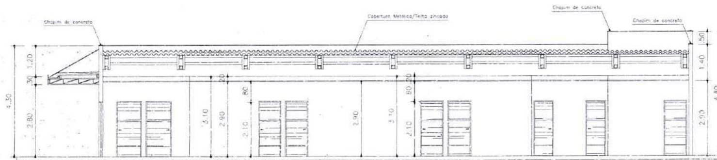
CORTE LONGITUDINAL ESCALA: 1/100
