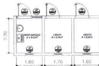
PLANTA BAIXA - ABRIGO DE LIXO ESCALA: 1/100
