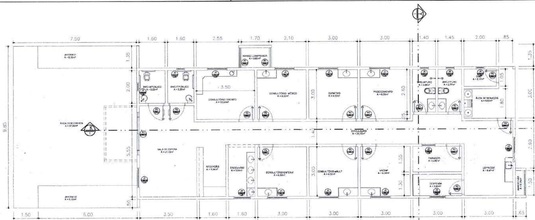
PLANTA BAIXA - EDIFICAÇÃO ESCALA: 1/100
